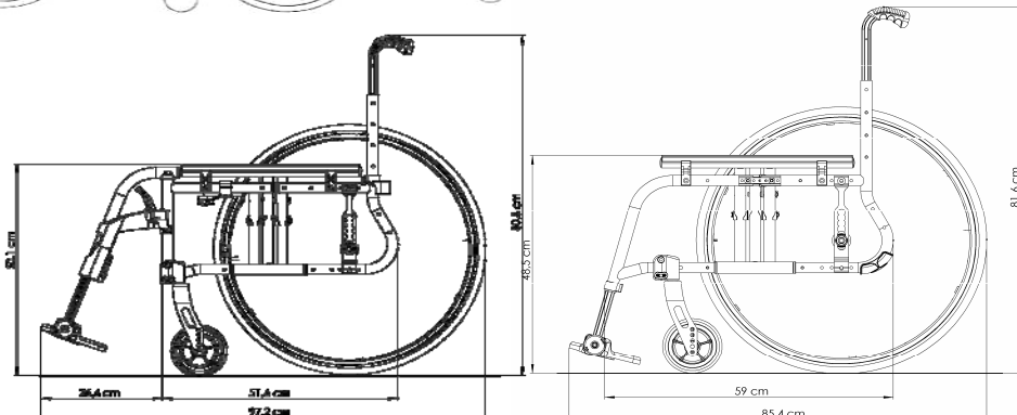
Especificaciones para sillas de 40 cm de anchura con ruedas traseras de 24"
